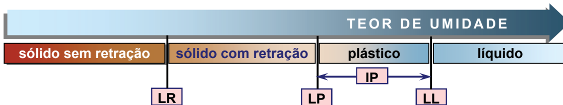
Figura 4 – Estado do solo, em função de seu teor de umidade
