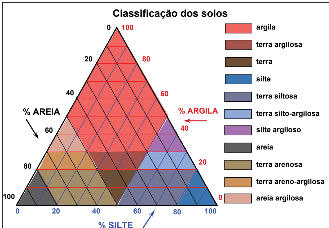
Figura 13 – Diagrama de classificação dos solos, pelo teste do vidro (adaptado de Aid at al (s/d) e Moran, 1984)
