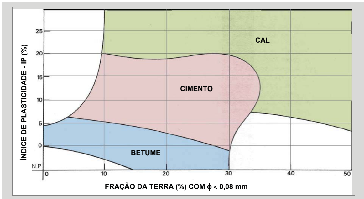
Figura 9 – Seleção do tipo de estabilizante, em função do Índice de Plasticidade (IP) e da granulometria da terra (adaptado de Houben & Guillaud, 1995)
