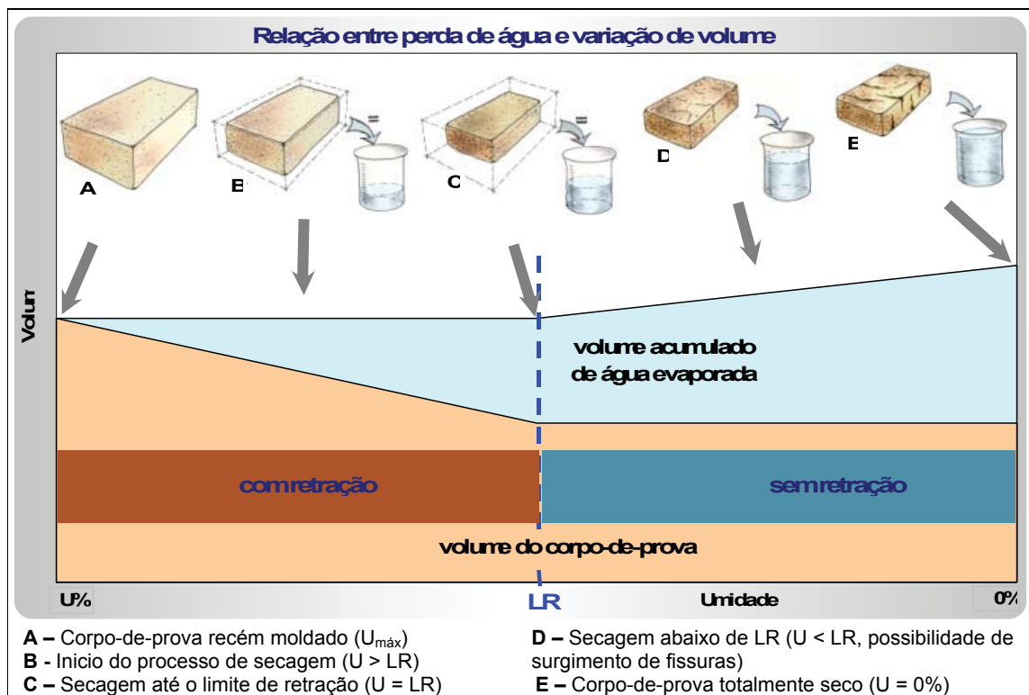
Figura 7 – Diagrama representativo da relação entre o limite de retração (LR) e as variações de volume, da terra e da água evaporada, durante o processo de secagem
