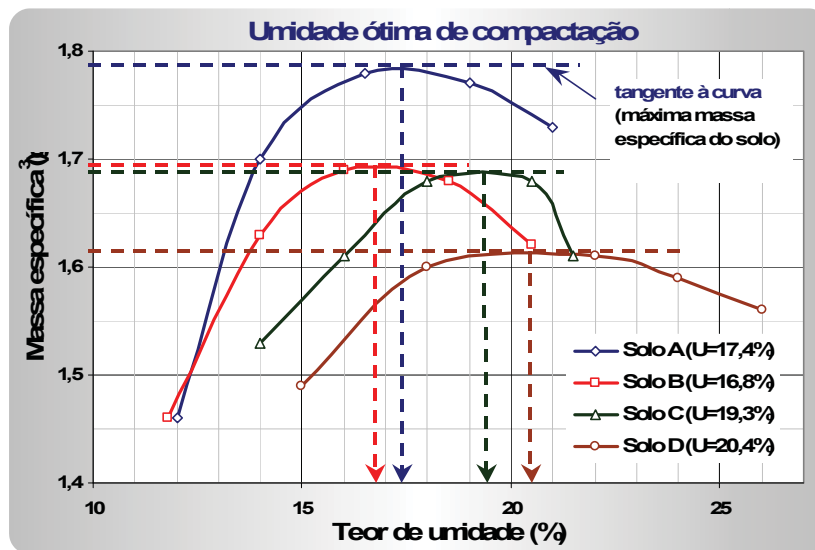
Figura 8 – Resultados de ensaios de compactação, para quatro diferentes tipos de solos
