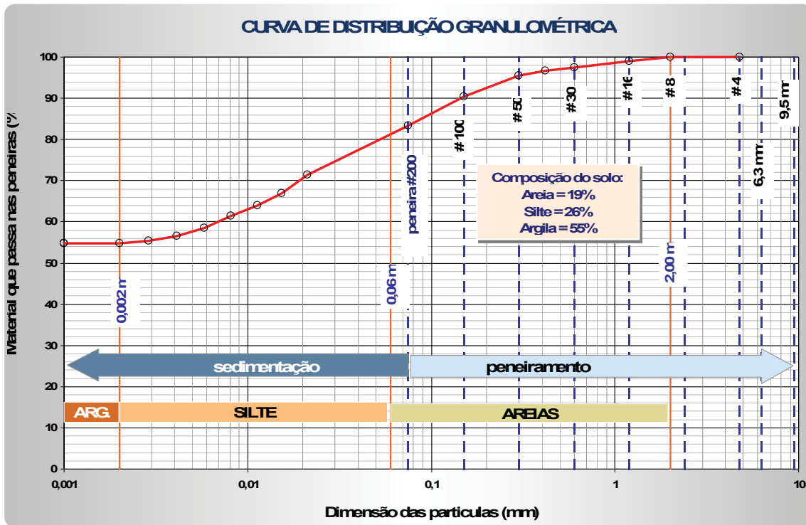
Figura 1 – Exemplo de curva de distribuição granulométrica, com indicação das frações que compõem o solo, além das faixas para ensaio de peneiramento e de sedimentação (adaptado de FARIA, 2002)
