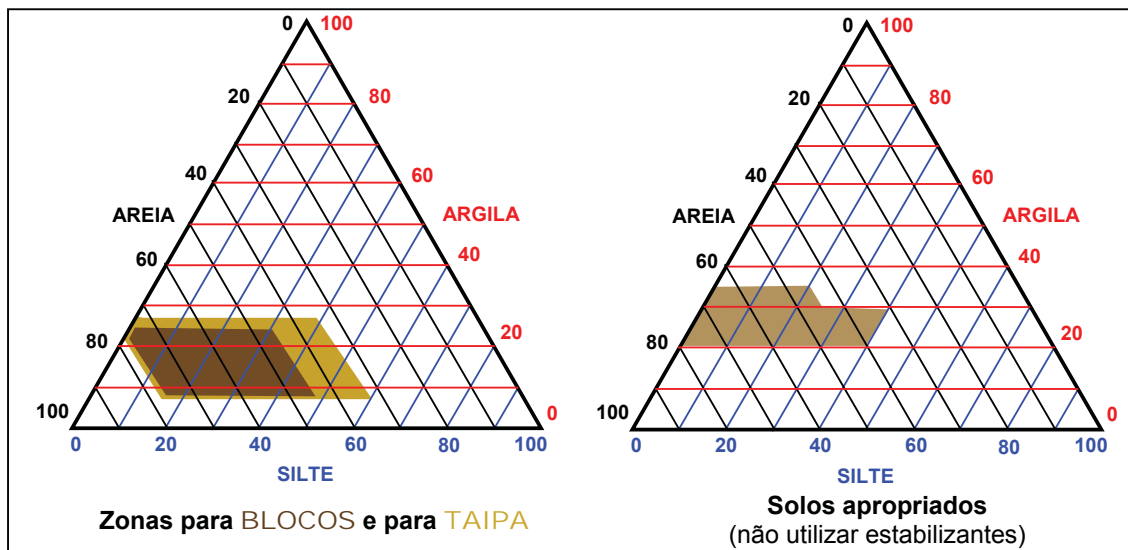
Figura 14 – Diagramas indicativos de uso da terra, pelo teste do vidro (adaptado de Aid at al (s/d) e Moran, 1984)
